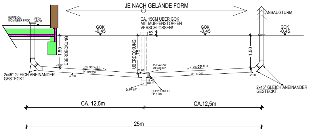
SCHNITT A-A M=1:50
