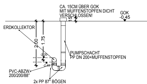
SCHNITT B-B M=1:50
